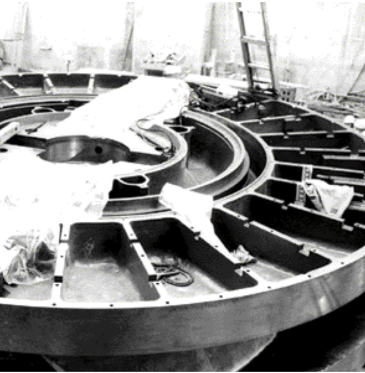
その巨大さゆえ輸送に困難を極めた2分割水車
