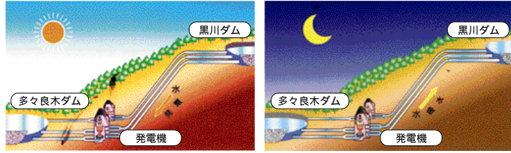
昼間 上部の黒川ダムから下部の多々良木ダムに水を落とすとして発電する。 夜間 ゆとりある深夜に火力・原子力発電所の電気を利用して、下のダムから水をくみ揚げて昼間に備える。
